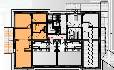
SCHÉMA PŮDORYSU OBJEKTU
